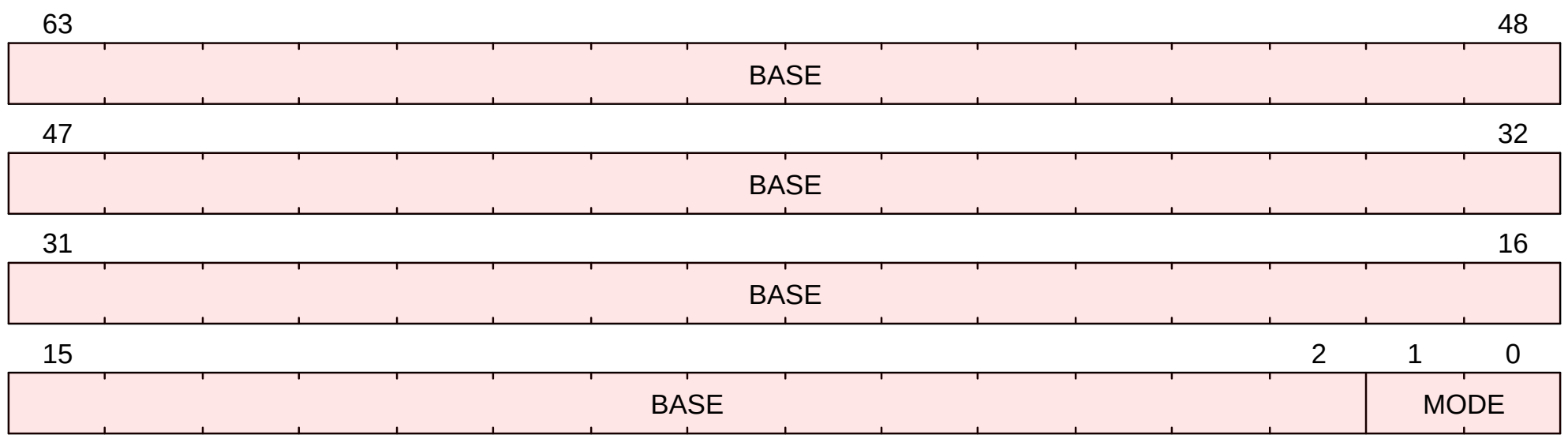
Figure 67. stvec format
