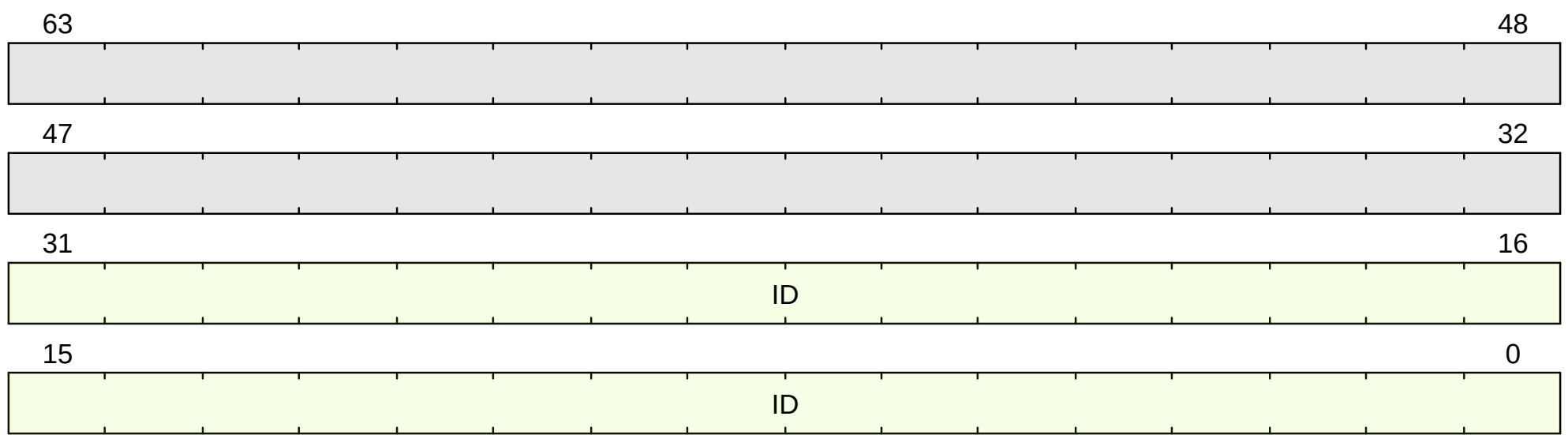
Figure 41. mhartid format
