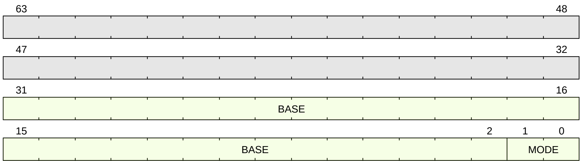
Figure 53. mtvec format
