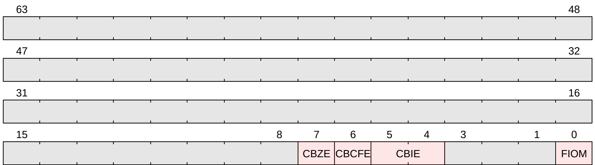
Figure 60. senvcfg format
