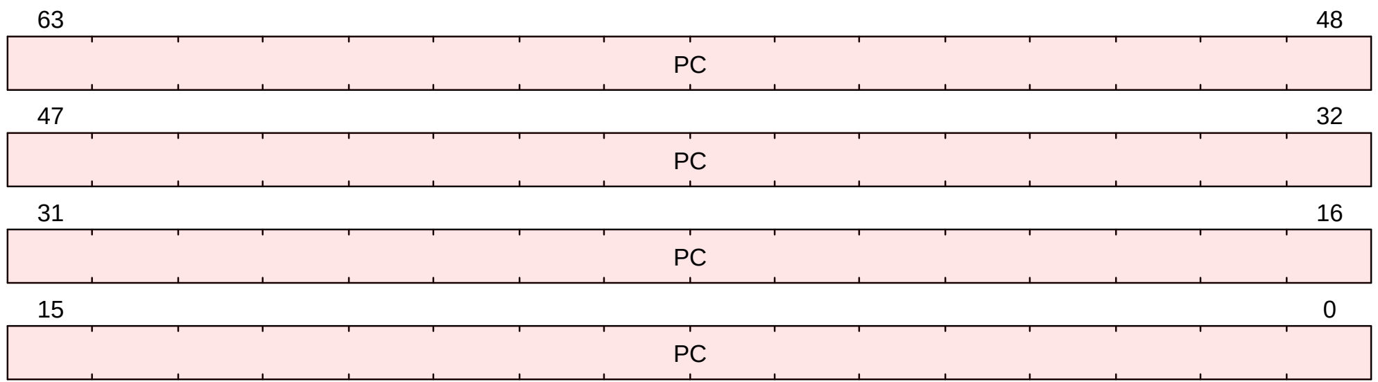
Figure 61. sepc format
