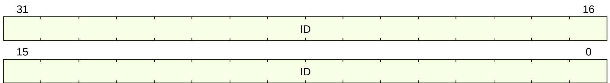
Figure 11. mhartid format
